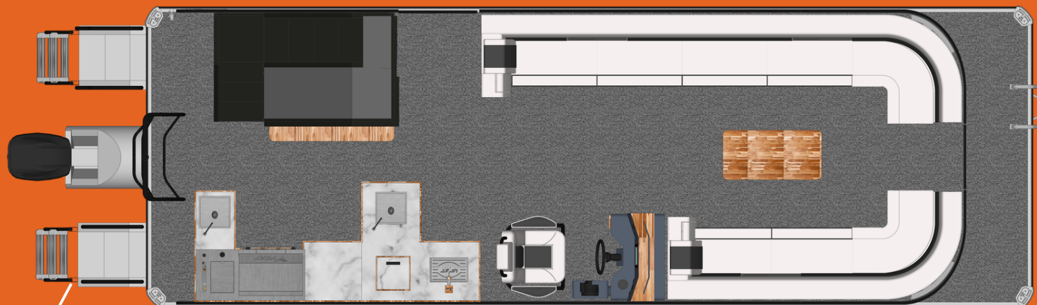
*Espaço gourmet ilustrado: V522 com adicional de choppeira
