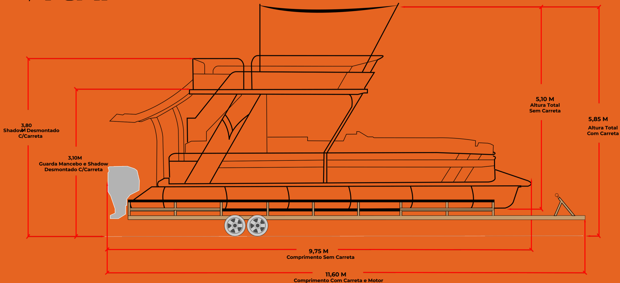
AURORA 900UP VISTA LATERAL
